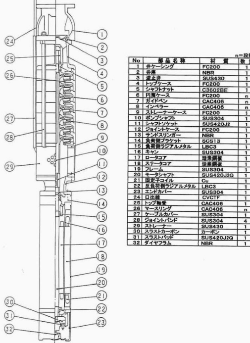
2号取水井戸ポンプ構造断面図
