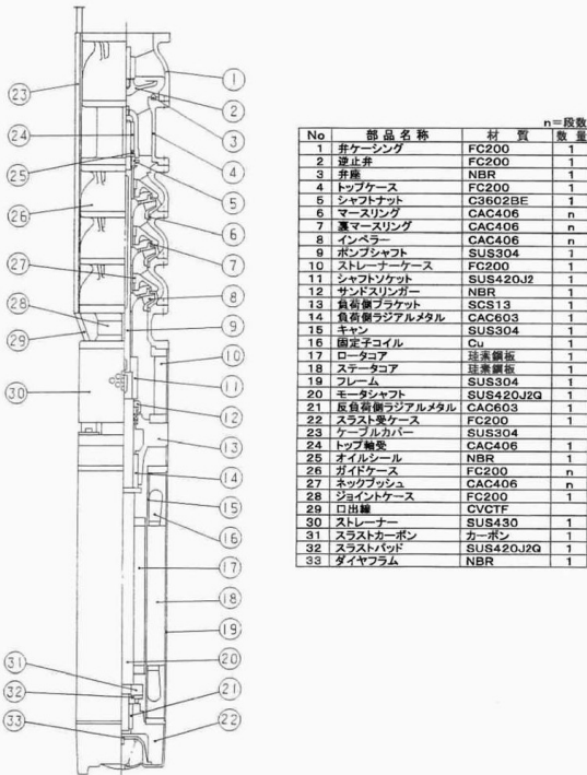
1号取水井戸ポンプ構造断面図
