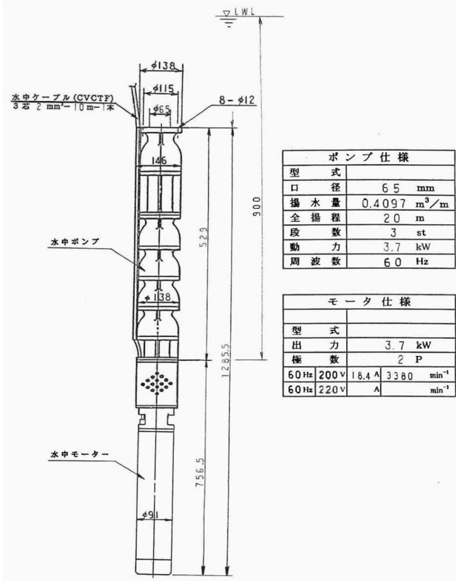
1号取水井戸ポンプ外径寸法図
