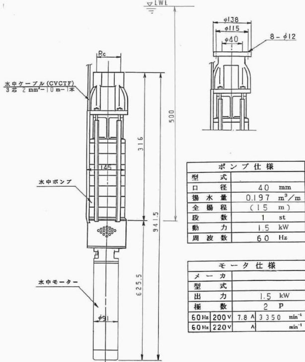
2号取水井戸ポンプ外径寸法図
